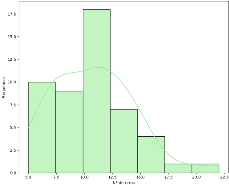
Histograma sobre Erros de Impressão
