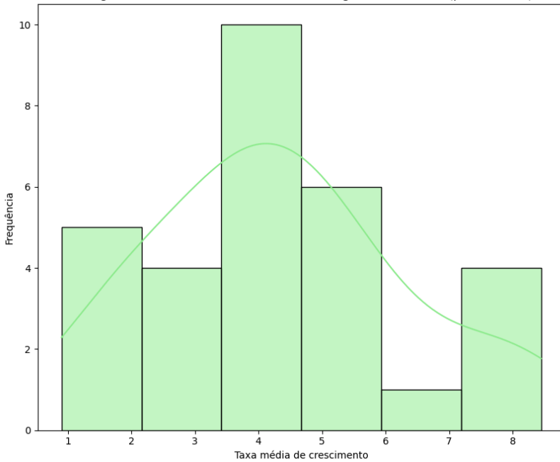
Histograma sobre Taxa média de crescimento geométrico anual (por 100 hab.)
